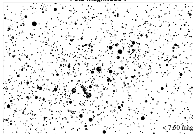
Peta Magnitudo 7
